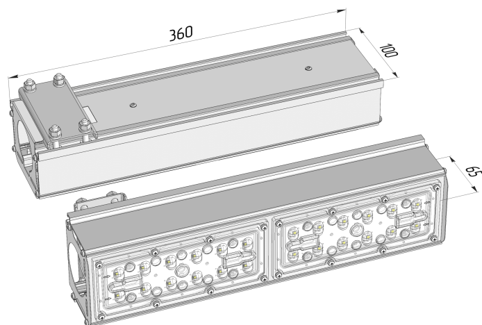
Габаритный чертёж
