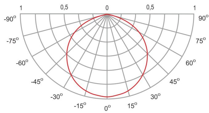
Диаграмма КСС типа Д (косинусная)
