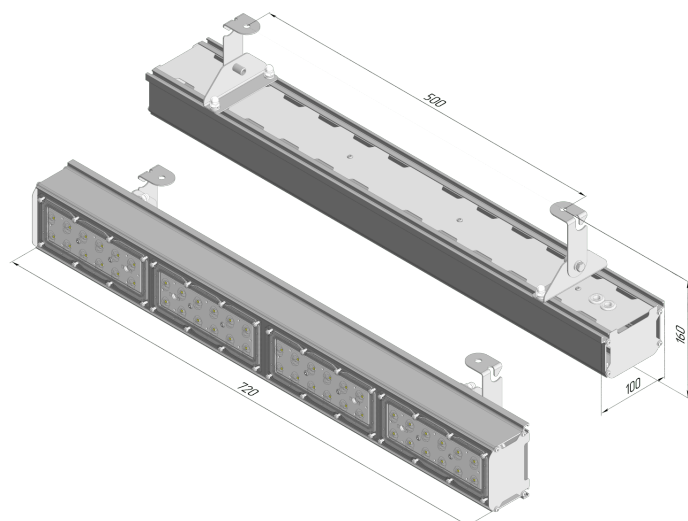
Габаритный чертёж
