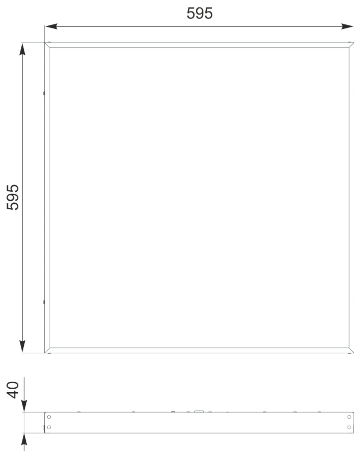
Габаритный чертёж
