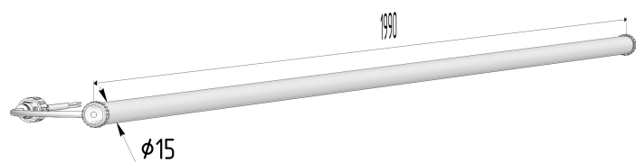
Габаритный чертёж
