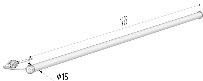
Габаритный чертёж
