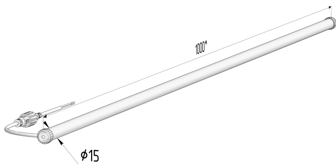
Габаритный чертёж
