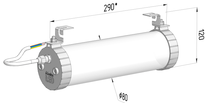
Габаритный чертёж
