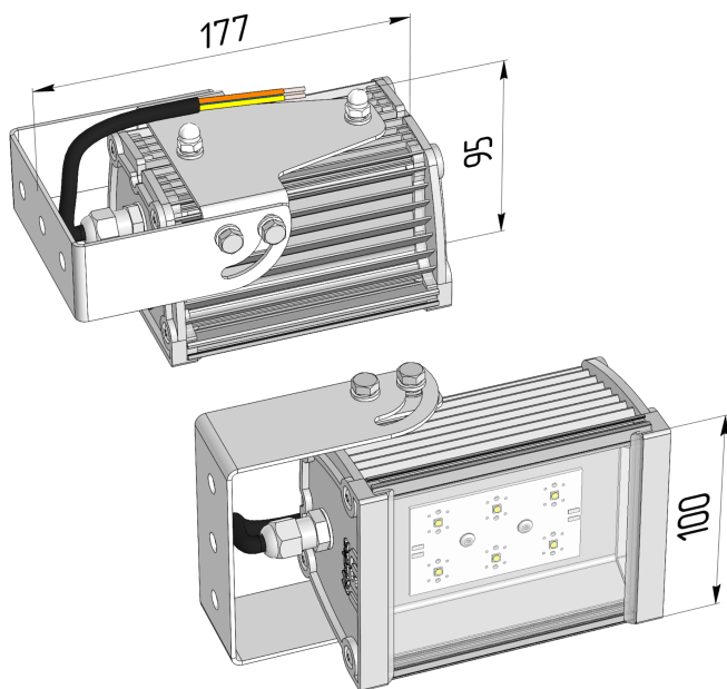
Габаритный чертёж
