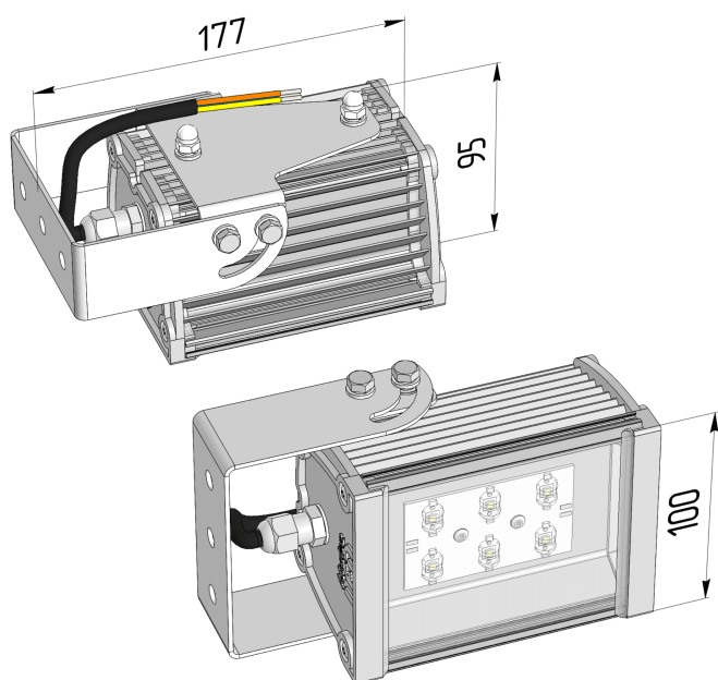
Габаритный чертёж
