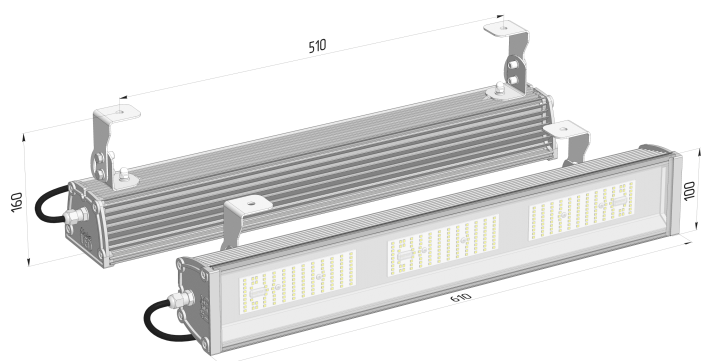
Габаритный чертёж
