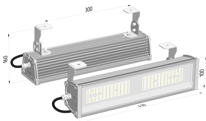
Габаритный чертёж
