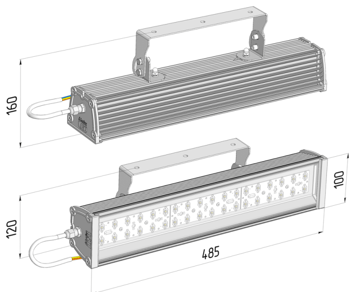
Габаритный чертёж
