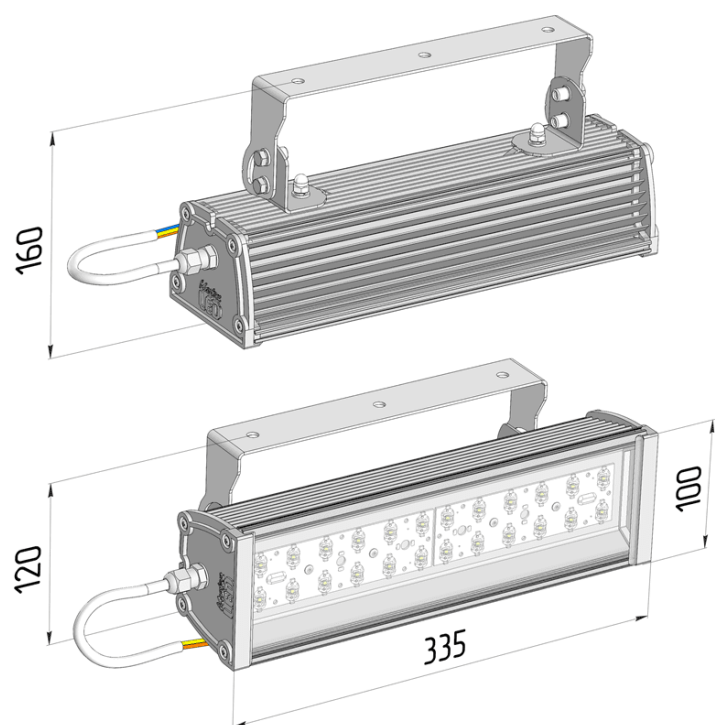
Габаритный чертёж
