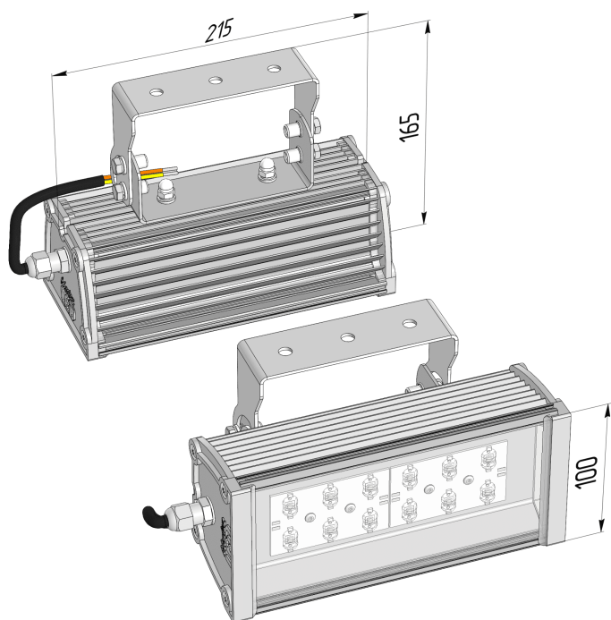
Габаритный чертёж
