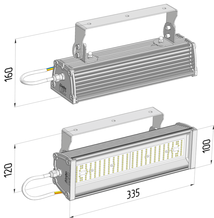
Габаритный чертёж
