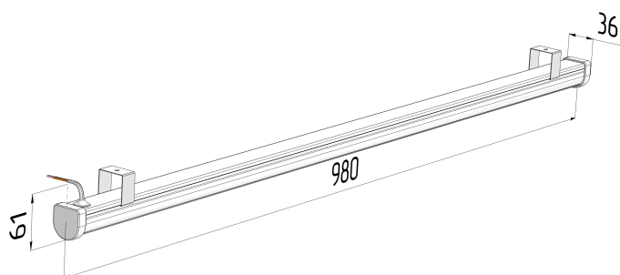
Габаритный чертёж
