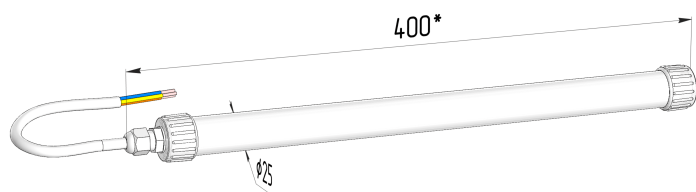
Габаритный чертёж
