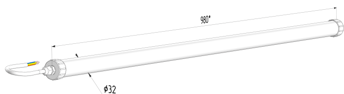
Габаритный чертёж
