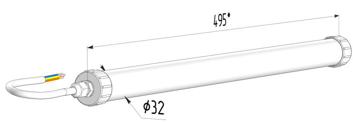
Габаритный чертёж
