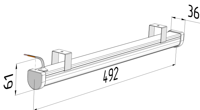
Габаритный чертёж
