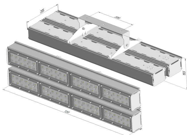
Габаритный чертёж
