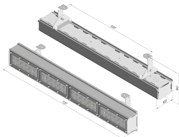
Габаритный чертёж
