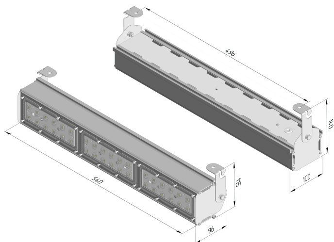
Габаритный чертёж
