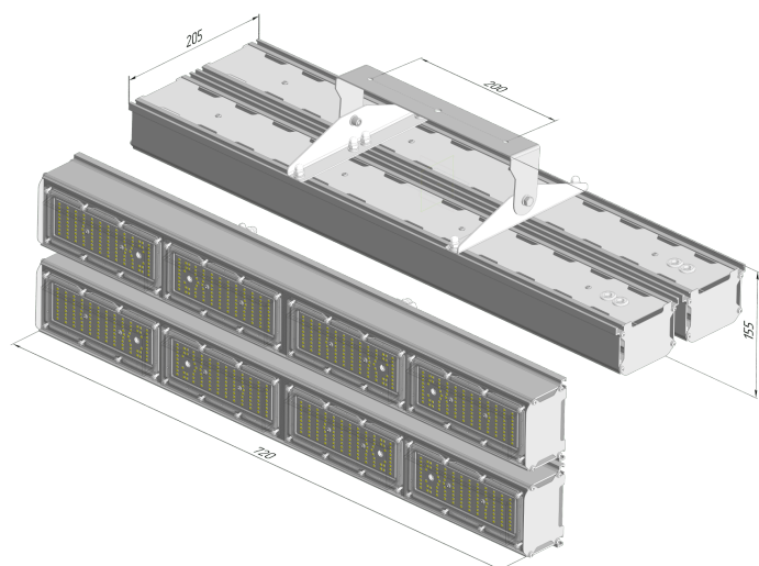
Габаритный чертёж
