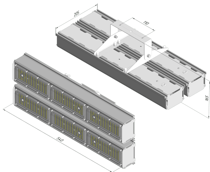
Габаритный чертёж
