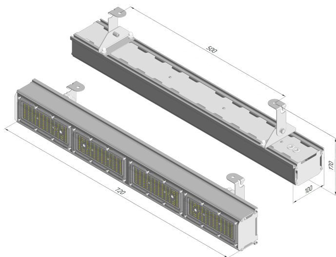
Габаритный чертёж
