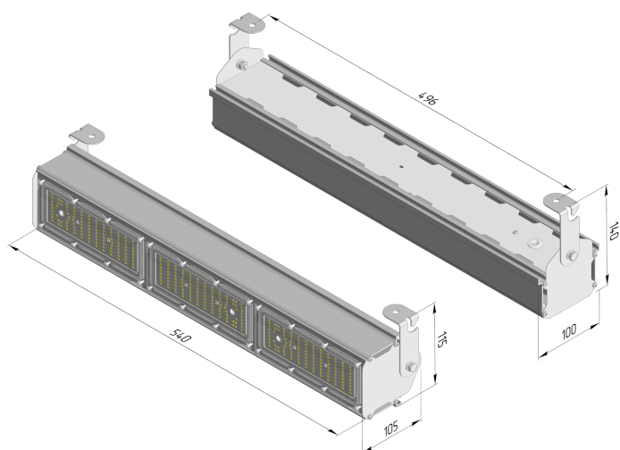
Габаритный чертёж
