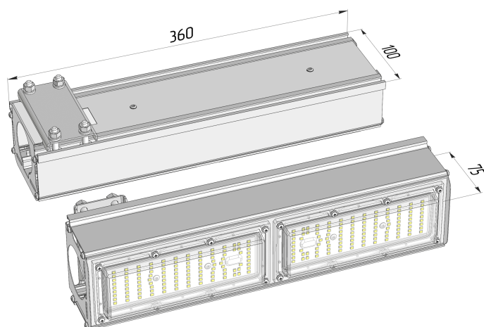
Габаритный чертёж
